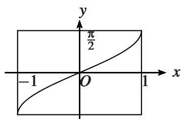
FIGURE 10 – Le graphe de \arcsin
