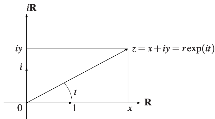
FIGURE 49 – Représentation graphique de \mathbb{C} .
