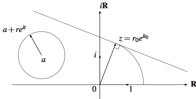
FIGURE 51 – Une droite et un cercle dans \mathbb{C}
