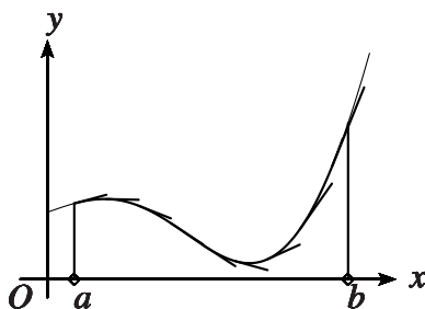
FIGURE 43 – Approximation d'une courbe par des segments de droites tangentes
