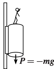
FIGURE 56 – Chute d'un corps
