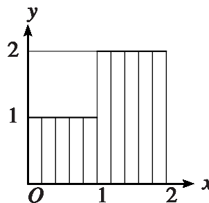
FIGURE 41 – Intégrale d'une fonction en escalier (deux marches)
