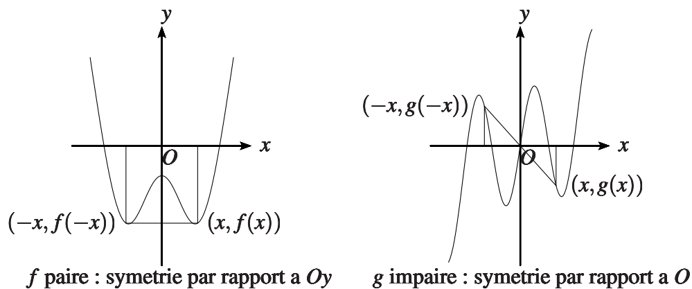
FIGURE 2 – Symétrie du graphe en fonction de la parité
