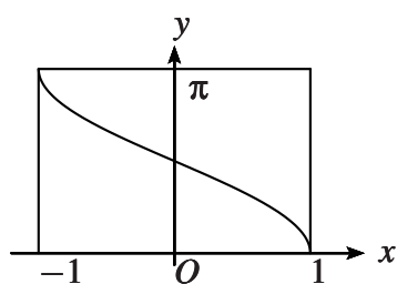
FIGURE 9 – Le graphe de \arccos
